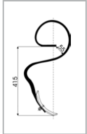
SFZ 32x10 Art.-Nr. 120 0250
