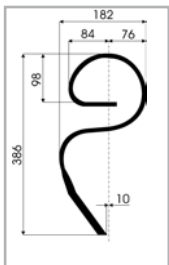
GEZ 25x8 Art.-Nr. 120 8822
