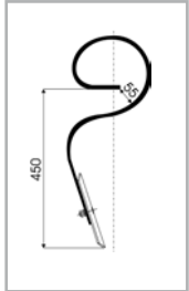
FZ 32x12 EH 450 mm Art.-Nr. 120 0245
