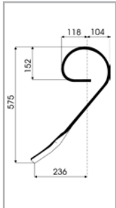
Schleppzinken 32x10 Art.-Nr. 120 9606
