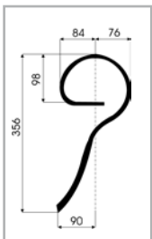
GEZ 25x8 Art.-Nr. 120 8830
