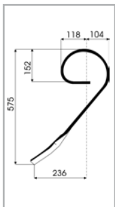
Тракторные зубья 32x10 Идент.-№ 120 9606
