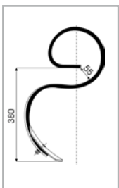
FZ 32x12 Идент.-№ 120 9028
