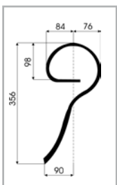
GEZ 25x8 Идент.-№ 120 8830
